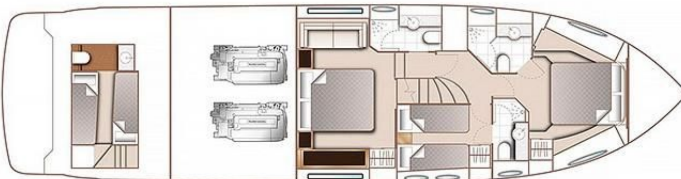
НИЖНЯЯ ПАЛУБА
